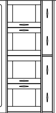
WITRYNA WYSOKA HAM2001 szer./głęb./wys. 100/40/188
