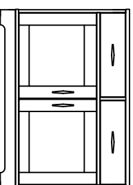
KOMODA 2D 2SZ HAM 2300 szer./głęb./wys. 118/45/85
