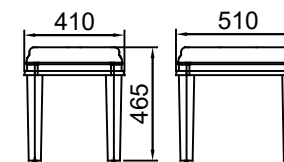
STÓLEK TOALETKI HEN0600
