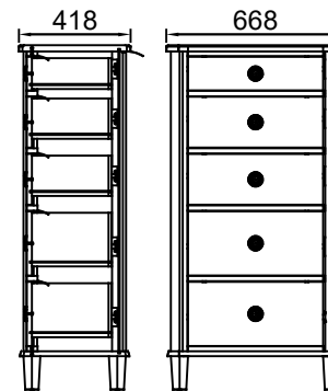
KOMODA WYSOKA 5SZ HEN0400
