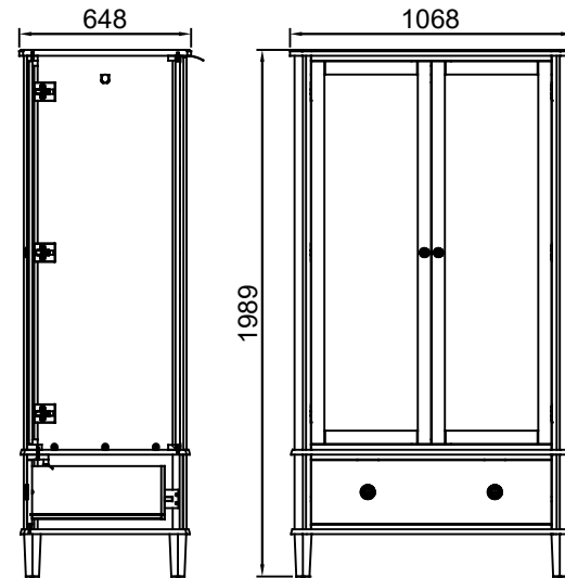
SZAFKA 2D 1SZ HEN1000
