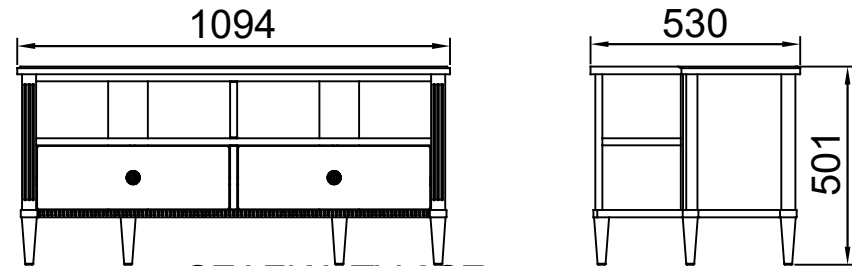
SZAFKA TV 2SZ. GUS2200
