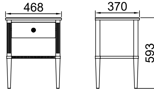
STOLIK 1SZ. GUS0101
