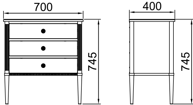
STOLIK 3SZ. GUS0102
