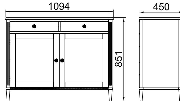
KREDENS 2D 2SZ GUS2300
