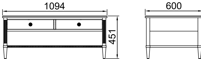
ŁAWA 2SZ. GUS2100
